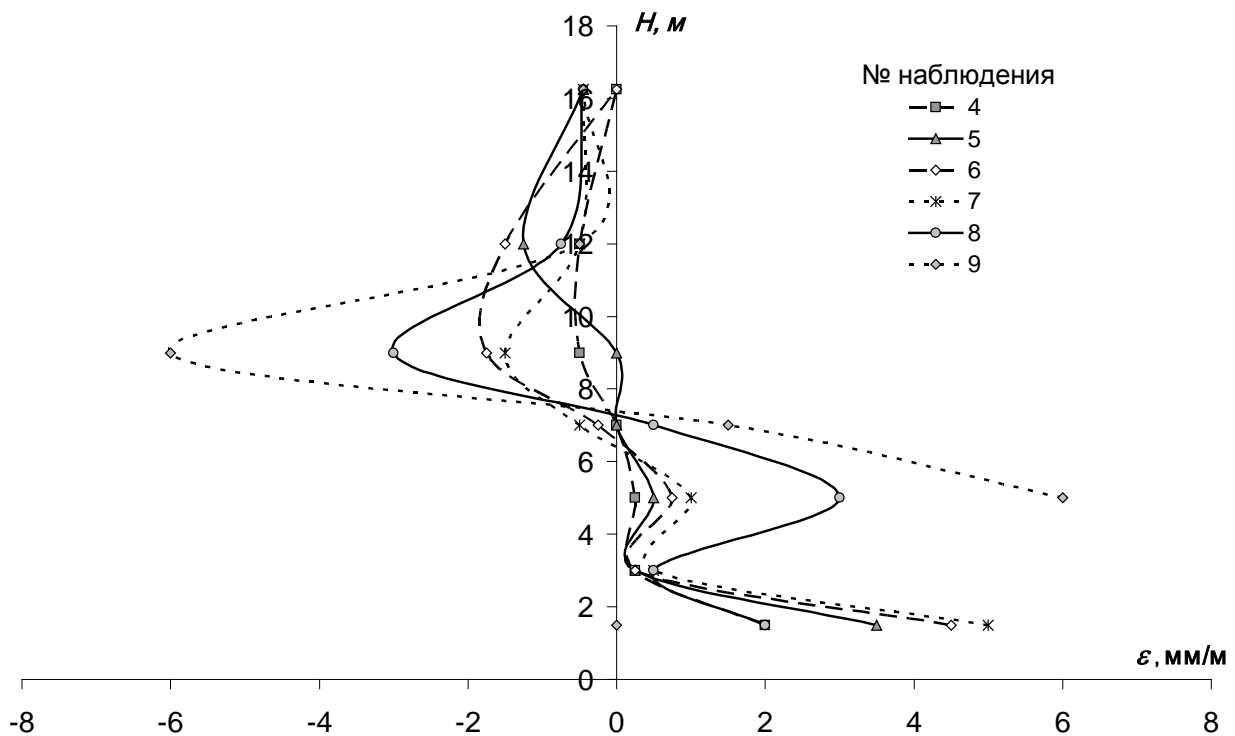
Рис. 3. Вертикальные деформации скважины на ПК 104+4
