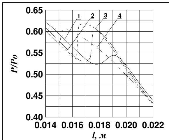
Рис. 1. Распределение давлений пара вдоль сопла для различных значений времени при неравновесном расширении в расширяющемся сопле: концентрация гетерогенных зародышей конденсации I_q = 0 1/кг 1 – t = 5,2212 \cdot 10^{-4} с; 2 – t = 5,7433 \cdot 10^{-4} с; 3 – t = 6,2654 \cdot 10^{-4} с; 4 – t = 6,7876 \cdot 10^{-4} с
