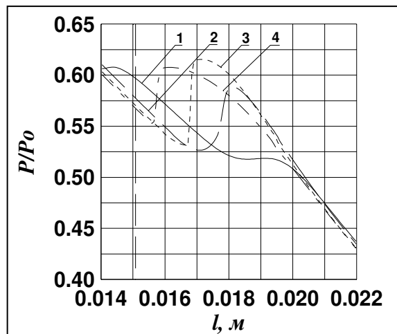
Рис. 2. Распределение давлений пара вдоль сопла для различных значений времени при неравновесном расширении в расширяющемся сопле: концентрация гетерогенных зародышей конденсации I_q = 1,0 \cdot 10^{13} 1/кг 1 – t = 5,2212 \cdot 10^{-4} с; 2 – t = 5,7433 \cdot 10^{-4} с; 3 – t = 6,2654 \cdot 10^{-4} с; 4 – t = 6,7876 \cdot 10^{-4} с
