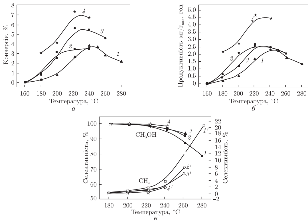
Рис. 1. Температурна залежність продуктивності каталізатора за метанолом (а), конверсії синтез-газу за вуглицем (б) та селективності (в): 1 — промисловий каталізатор у стаціонарному шарі; 2–4 — механоактивований каталізатор у віброрежимі ( f = 5 Гц): нанесений на кульки з однорідною гладкою (2) і неоднорідною (3) поверхнею; нанесений на кульки з однорідною поверхнею у присутності 0,1% добавки каталізатора (4) ( P = 0,1 МПа, U = 11000 год -1 )
