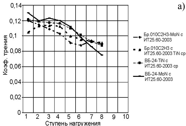
Рис. 4. Зависимость коэффициента трения от нагрузки для пар трения “сталь с покрытием – бронза”.
