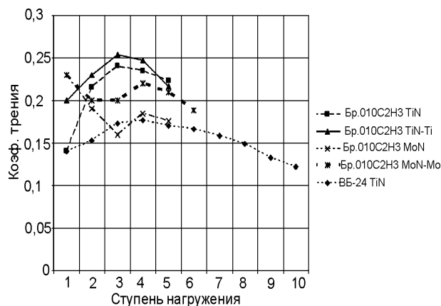
Рис. 4. Зависимость коэффициента трения от нагрузки для пар трения “сталь с покрытием – бронза”.
