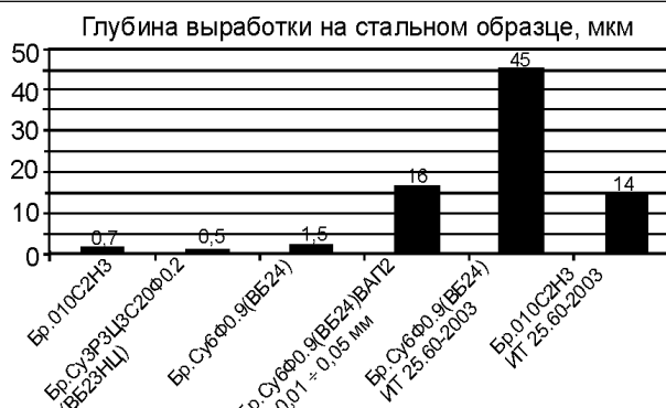
Рис. 2. Гистограмма износа образцов без покрытия.
