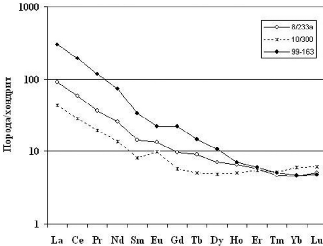
Рис. 2. Распределение РЗЭ для эндербитов и тоналитов. Нормировано на хондрит [12]
