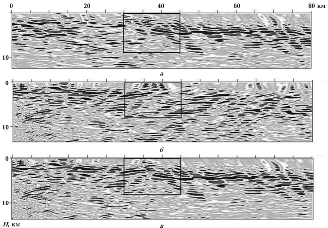
Рис. 5. Формирование изображение отдельной детали строения преломляющей границы: а и б — изображения, полученное для пункта возбуждения, расположенного справа ( а ) и слева ( б ) от нарушения; в — результирующее изображение нарушения.
