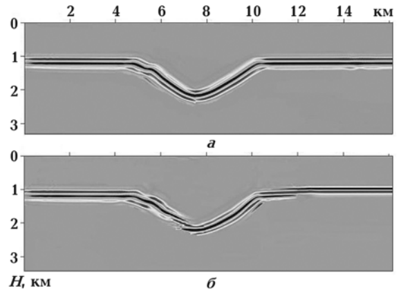
Рис. 3. Миграционные изображения преломляющей границы, полученные: а — по смоделированным волновым полям рис. 1, д, е для скоростной модели, представленной на рис. 2, б; б — по смоделированным волновым полям рис. 1, в, г для скоростной модели, представленной на рис. 2, а.
