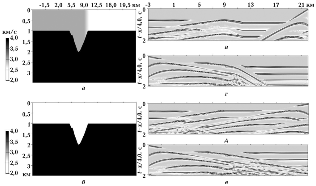
Рис. 2. Исследование влияния горизонтального градиента скорости в покрывающем слое на характер волнового поля: а — скоростная модель среды с горизонтальным градиентом скорости в покрывающем слое; б — скоростная модель среды с постоянной скоростью в покрывающем слое; смоделированные поля для встречных пунктов возбуждения, расположенных на -3 км и 22 км профиля со скоростью редукции 4 км/с: в и г — для модели а ; д и е — для модели б .
