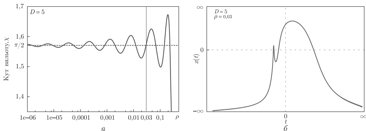
Рис. 3. Залежність кута вильйоту частинки від прицільного параметра в потенціалі \tilde{U}(x, y) за умови \chi_0 = 0 (а) та залежність x координати частинки при розсіянні з прицільним параметром \rho = 0,03 (б)
