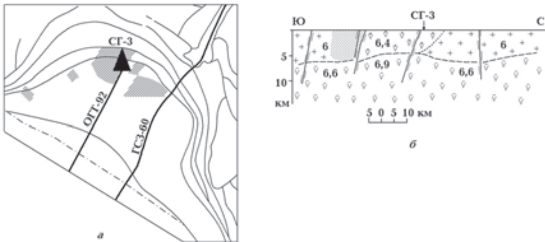
Рис. 2. Схема расположения профилей ОГТ-92, ГСЗ-60 (а) и предварительный сейсмический разрез ГСЗ-60 (б) [Литвиненко, 1963].
