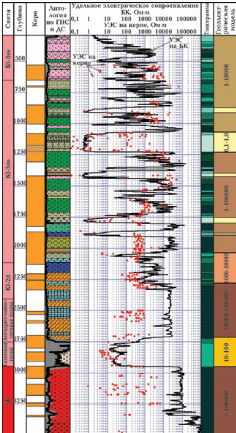
Рис. 10. Геоэлектрическая модель ОПС [Онежская ..., 2011].
