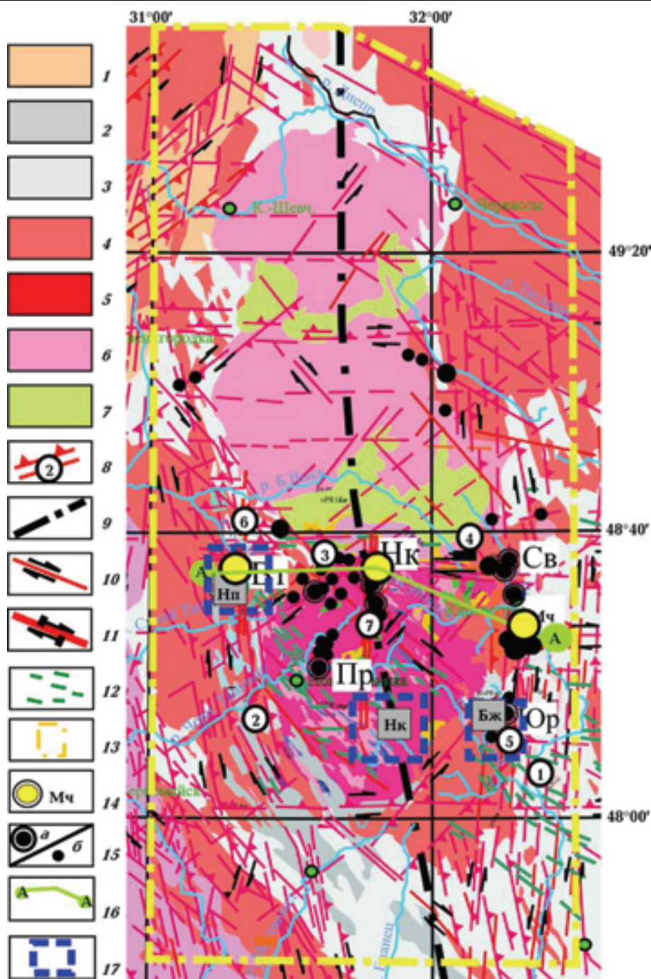
Рис. 1. Схема геологического строения Кировоградского рудного района: 1—5 — серии и комплексы (1 — росинско-тикичская (AR 3 ); звенигородский, гайсинский (PR 1 -I); ингуло-ингулецкая (PR 1 -I); 2 — родионовская, спасовская свиты; 3 — рошаховская, чечелевская свиты; 4 — кировоградский, уманский, ставищанский (PR 1 -I); 5 — новоукраинский (PR 1 -I); корсунь-новомиргородский (PR 1 -II)); 6 — рапаквивидные границы, 7 — габбро-анортозиты; 8 — эшелонированные сколы (сместители) зон разломов, берг-штрихи указывают направление падения; цифры в кружках — зоны разломов (1 — Западно-Ингулецкая, 2 —Звенигородско-Братская, 3 — Субботско-Мошоринская, 4 — Лелековская, 5 — Кировоградская, 6 — Первомайская); 9 — трансрегиональный тектонический шов Херсон — Смоленск; кинематические знаки для зон разломов : 10 — правый сдвиг и левый сдвиг, 11 — сбросо-сдвиг и взбросо-сдвиг; 12 — дайки, 13 — контур КРР; 14 — урановые месторождения, изученные тектонофизическими методами (Мч — Мичуринское, Нк — Новокопанинское, Вт — Ватутинское); 15 — a — другие месторождения (Св — Севериновское, Пр — Партизанское, Юр — Юрьевское); b — рудопоявления; 16 — линия разреза, представлено на рис. 6; 17 — контуры участков детальных тектонофизических исследований.
