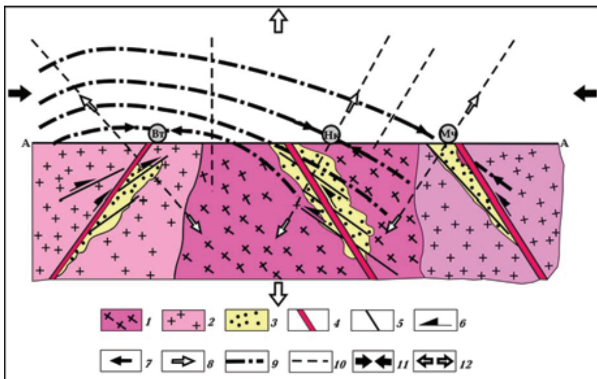
Рис. 6. Схематический разрез КРР по линии, соединяющей Ватутинское (Вт), Новоконстантиновское (Нк) и Мичуринское (Мч) месторождения, а также схема напряженного состояния КРР во время формирования урановорудных полей: 1 — новоукраинские трахитоидные граниты, 2 — кировоградские порфиоровидные граниты, 3 — рудные и рудовмещающие комплексы (ураноносные натровые метасоматиты), 4 — основные сместители (L-сколы), 5 — R-сколы и трещины отрыва, 6 — направление взбросов и надвигов; 7, 8 — главные оси нормальных напряжений (7 — сжатия ( \sigma_1 ), 8 — растяжения ( \sigma_3 )); 9, 10 — траектории (9 — \sigma_1 , 10 — \sigma_3 ); 11, 12 — генеральные направления (11 — сжатия КРР, 12 — растяжения КРР).
