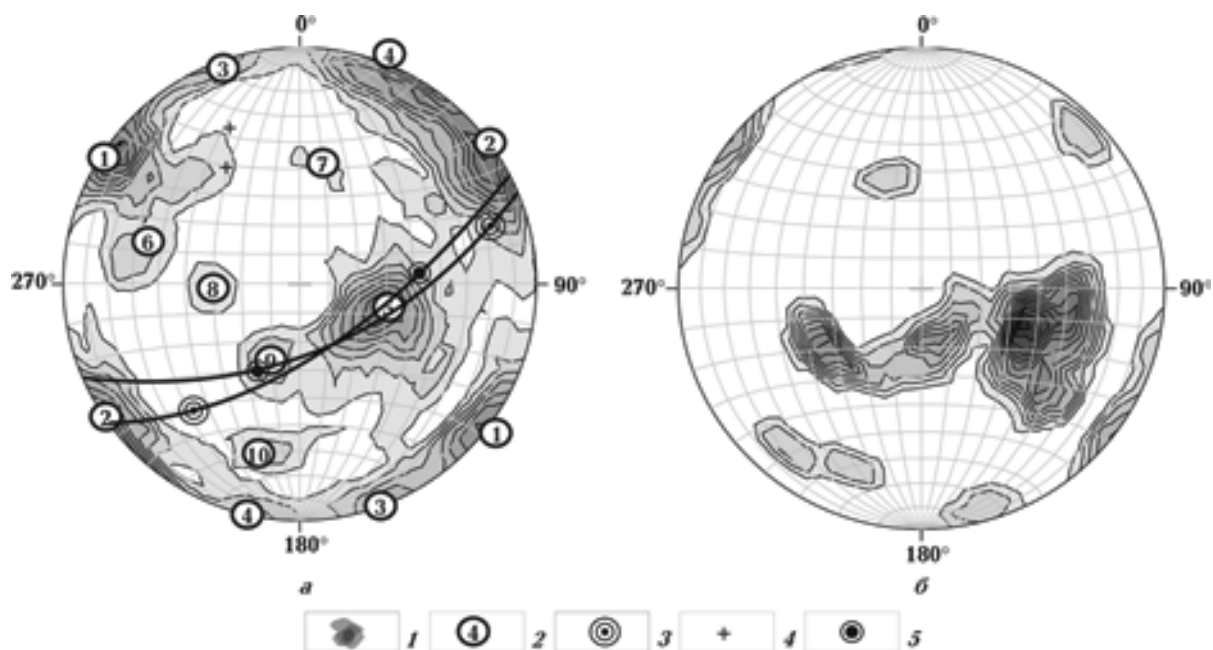
Рис. 2. Результаты тектонофизических исследований в пределах Бобринецко-Жевановской зоны скальвания на участке южнее с. Жевановка: а — стереограмма основных систем разрывов и полей напряжений (1 — изолинии концентрации полюсов разрывов; 2 — номера максимумов концентрации; 3—5 — оси главных нормальных напряжений (3 — \sigma_1 , 4 — \sigma_2 , 5 — \sigma_3 ); б — стереограмма изолиний концентрации полюсов полосчатости и линейности в кировоградских гранитах.
