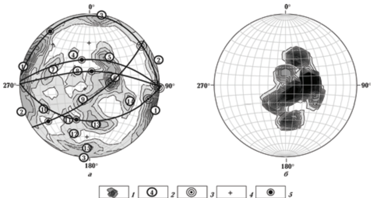
Рис. 4. Результаты тектонофизических исследований в пределах Новокопстантиновской зоны скальвания на участке севернее пос. Ровное: а — стереограмма основных систем разрывов и полей напряжений; б — стереограмма изолиний концентрации полюсов полосчатости и линейности в новоукраинских гранитах. Условные обозначения см. на рис. 2.
