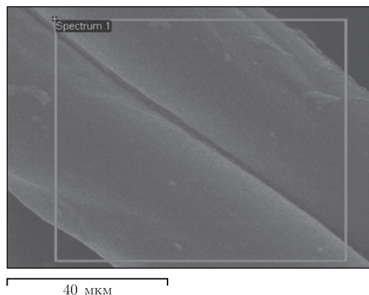
Рис. 2. СЭМ-изображение поверхности композитных волокон с осажденным слоем ГОЖ
