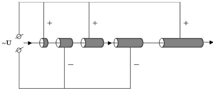
Рис. 1. Схема лінійного прискорювача
