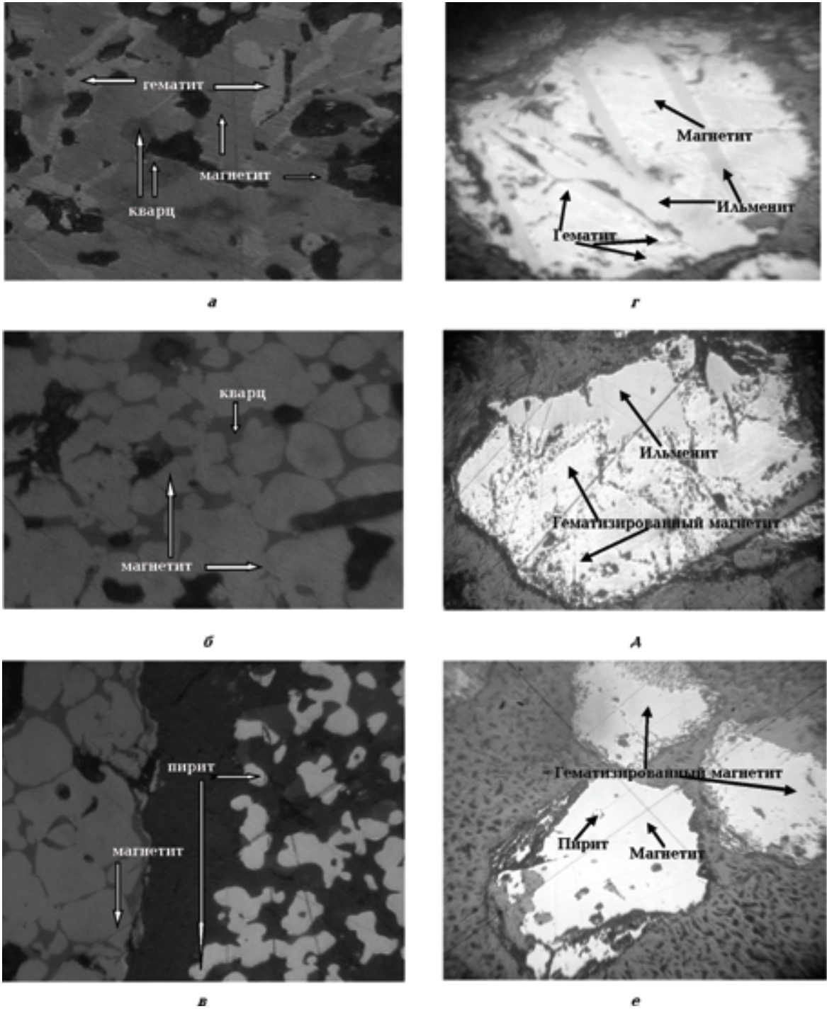
Рис. 1. Минералогический состав искусственного аналога природного магнитного песка (а, б, в) и необогащенного магнитного песка с берега Красного моря (г, д, е) на основании анализа аншлифов. Образцы с наличием: а — магнетита, гематита, кварца (увеличение \times 500 ); б — магнетита и кварца ( \times 500 ); в — магнетита и пирита ( \times 125 ); г — магнетита, гематита и ламелей ильменита ( \times 300 ); д — ильменита и гематизированного магнетита ( \times 120 ); е — магнетита, гематизированного магнетита и зерна пирита ( \times 120 ).
