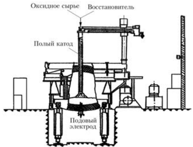
Рис. 2. Плазменная печь для восстановительной плавки оксидного сырья
