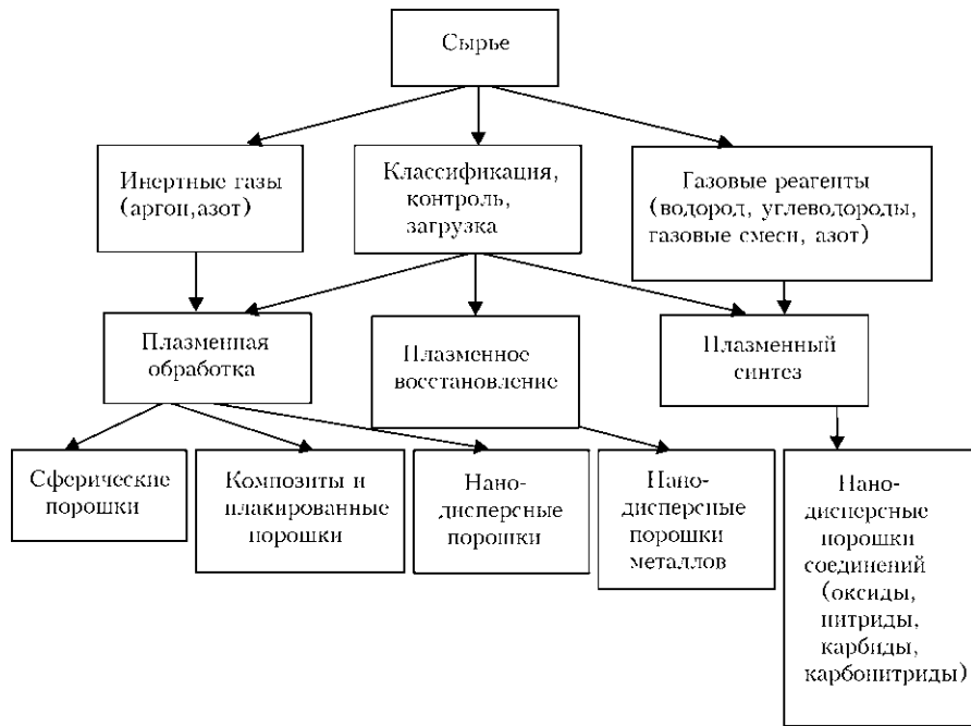
Рис. 4. Схема плазменной технологии производства порошков
