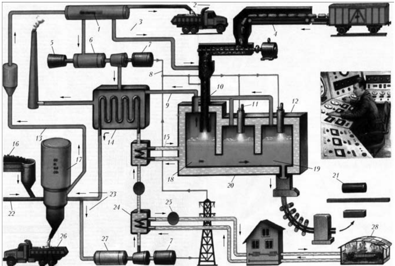
Рис. 10. Схема прогнозируемой металлургии будущего: 1 – газоочистка; 2 – сера; 3 – восстановительный газ; 4 – железорудный концентрат; 5 – компрессор; 6 – газовая турбина; 7 – генератор; 8 – подача электроэнергии; 9 – отработанный газ; 10 – плазмотрон (восстановление); 11 – плазмотрон (очистка); 12 – плазмотрон (легирование); 13 – газификатор; 14 – бойлер; 15 – вода; 16 – уголь; 17 – \text{CO} , \text{H}_2 , \text{H}_2\text{O} , \text{CO}_2 ; 18 – железо; 19 – сталь; 20 – металлургический блок; 21 – прокат; 22 – кислород; 23 – пар; 22 – теплообменник; 25 – насос; 26 – зола; 27 – паровая турбина; 28 – теплица
