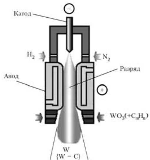
Рис. 6. Принципиальная схема получения нанопорошков вольфрама и {W-C} в струе термической плазмы дугового разряда
