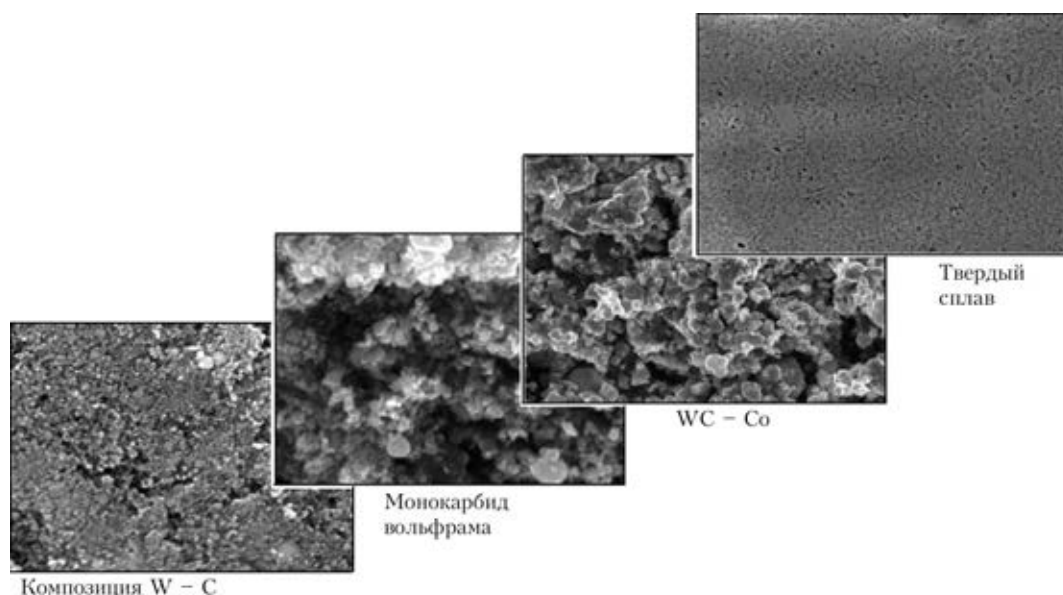
Рис. 7. Стадии получения наноструктурного твердого сплава
