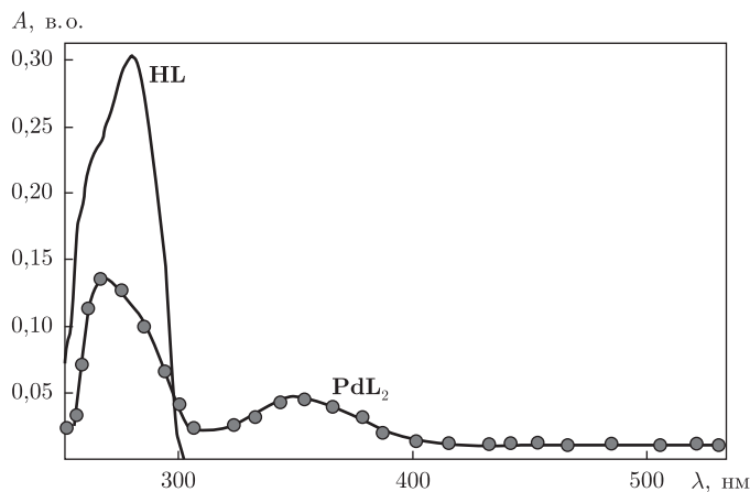
Рис. 2. Електронні спектри поглинання комплексу PdL 2 та ліганду HL
