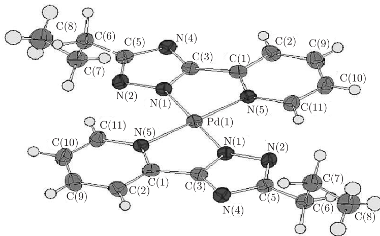
Рис. 1. Молекулярна будова комплексу складу \text{PdL}_2
