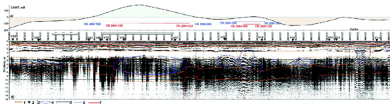
Рис. 3. Вертикальный георадарный разрез вдоль дороги (точки ВЭРЗ 23–11): а – график поля СКИП; б – георадарный разрез; 1 – литологические границы; 2 – пункты зондирования ВЭРЗ; 3 – тектонические нарушения аргиллит-алевролитовой толщи; 4 – зоны повышенной фильтрации грунтовых вод; 5 – подпорные стены; 6 – увлажненные зоны; 7 – оползнеопасные участки
