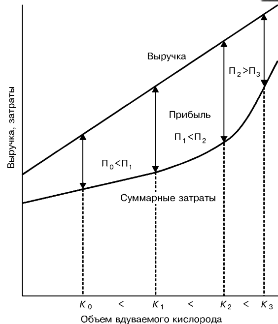
Рис. 2. Зависимость прибыли от интенсивности продувки
