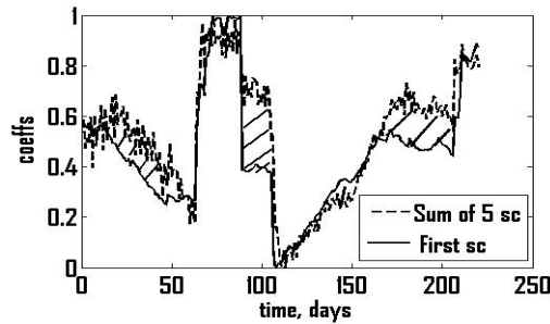
Рис. 2. Схематична ілюстрація ділянок (заштриховані) необхідних для розрахунку індексу фрактальності (штриховою лінією позначене середнє значення суми міри на 5 масштабах, суцільною – значення показника на першому масштабі, приведені після нормалізації)
