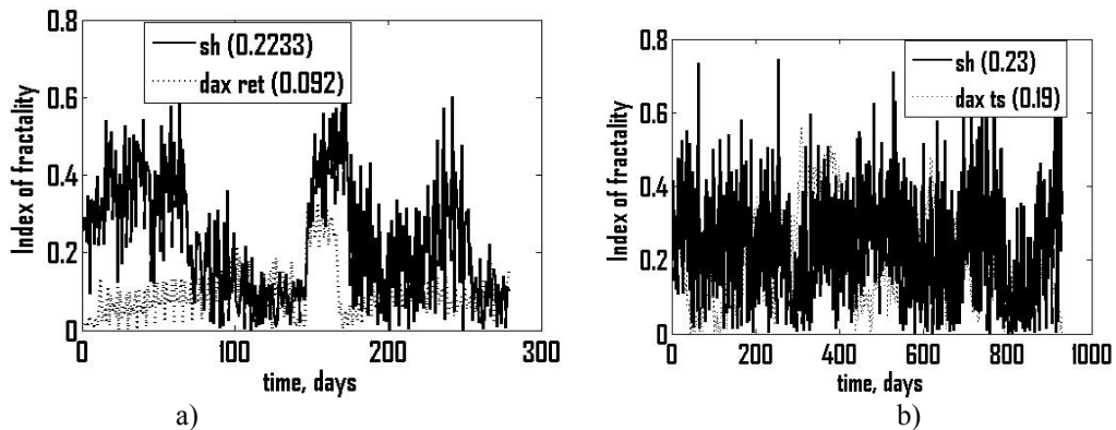
Рис. 3. Індекс фрактальності для а) стаціонарного часового ряду фондового індексу Німеччини (dax ret) та перемішаного ряду (sh), б) для нестаціонарного часового ряду (dax ts) та перемішаного ряду (sh), в дужках вказане середнє значення для всього ряду
