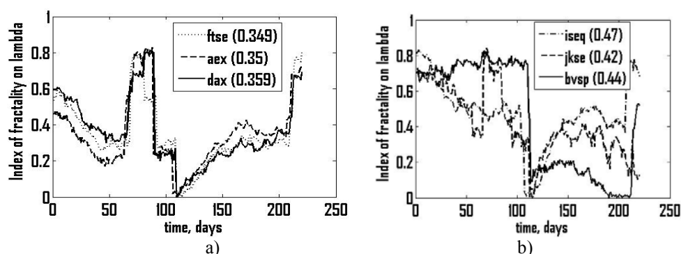
Рис. 4. Індекс фрактальності а) для розвинених країн (ftse – фондовий індекс Англії, aex – Нідерландів, dax - Німеччини), б) для країн, які розвиваються (iseq – фондовий індекс Ірландії, jkse – Індонезії, bvsp - Бразилії), в дужках вказане середнє значення для всього ряду
