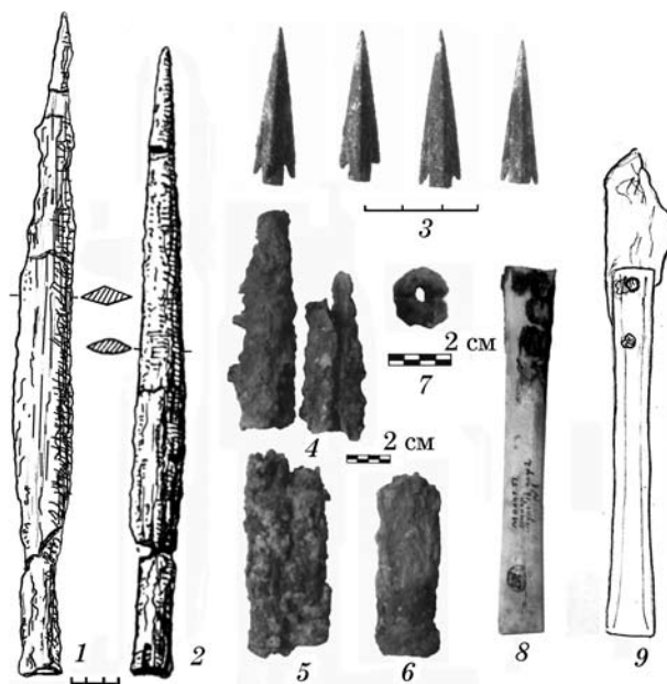
Рис. 7. Находки из погребения: 1—2 — наконечники копий; 3 — наконечники стрел; 4, 6 — втулки копий; 5 — подточки; 7 — ворварка; 8—9 — нож (фото и рисунок)
