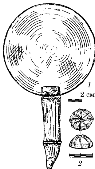
Рис. 8. Находки из погребения: 1 — зеркало с деревянной ручкой; 2 — пуля свинцовая
