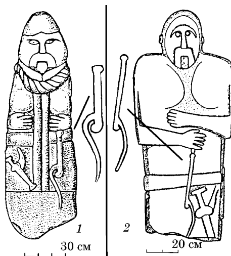
Рис. 11. Изображения нагаек на каменных изваяниях: 1 — Ольховчик; 2 — Таттарка
