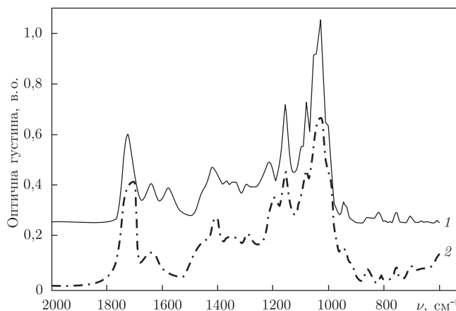
Рис. 1. ІЧ-спектри \beta -ЦД та його похідних: 1 — \beta -ЦД-(МА) 5 ; 2 — \beta -ЦД-(Ак) 7
