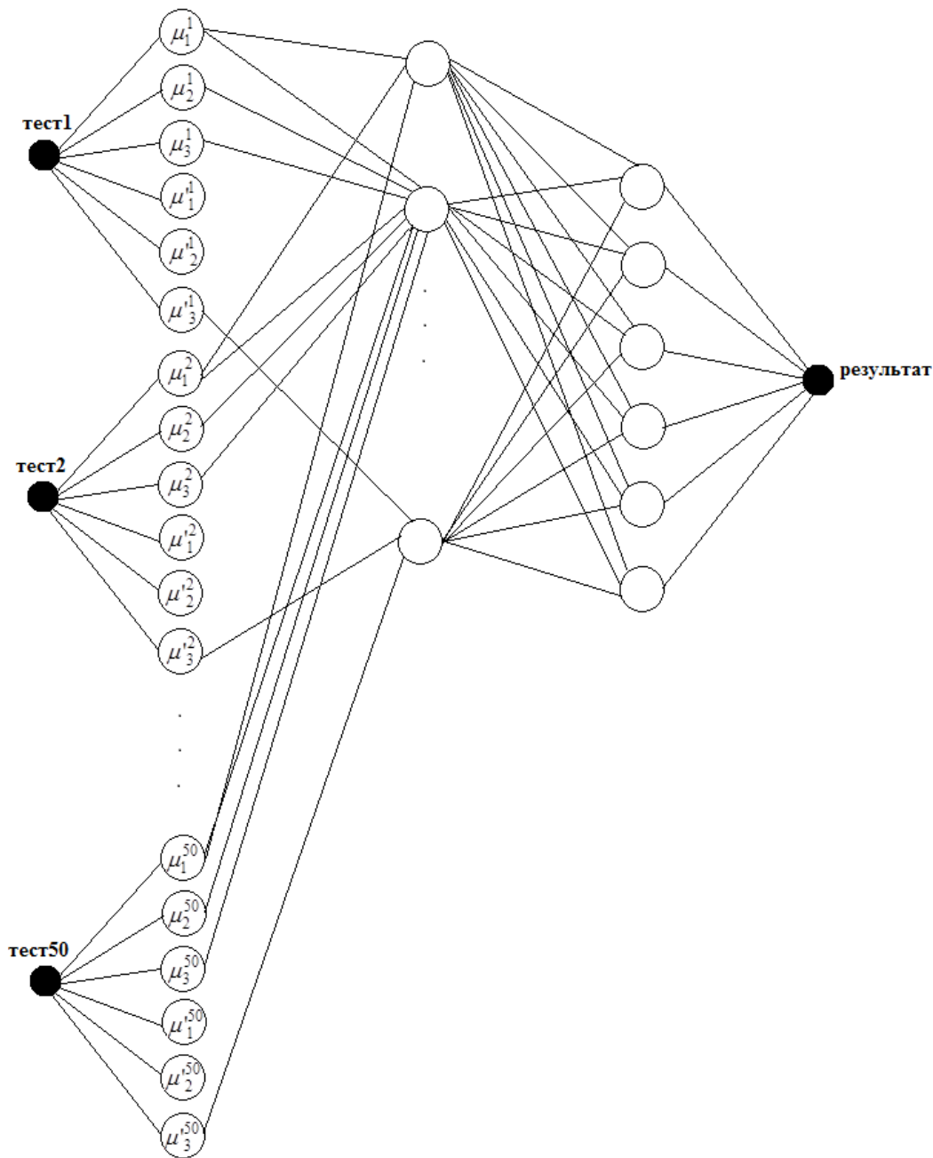
Рисунок 1 – Структура нечіткої нейромережі для оцінювання відповідності ПЗ критичного застосування вимогам
