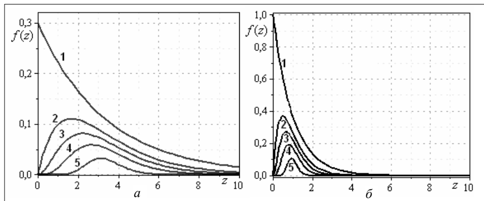
Рис. 1. Густина ерлангівського розподілу для різних значень параметра n при \mu = 0,3 (а) та \mu = 1 (б). Криві 1–5 відповідають значенням n = 1, 2, 3, 4, 5
