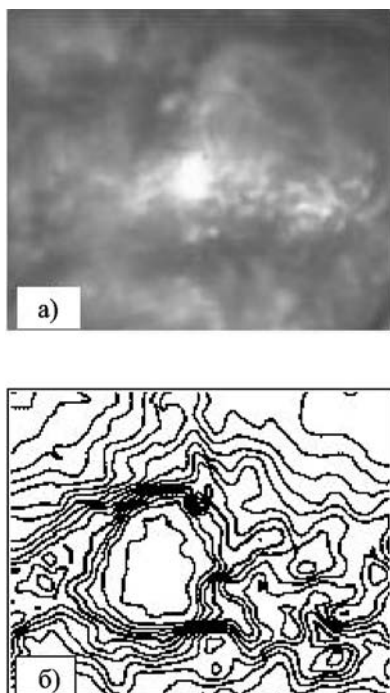
Рис. 3. Излучение области вспышки M8.2 в линии 195 Å 10.04.2002 г. в 12:13 UT: а) – тональное изображение; б) – увеличенное оконтурненное изображение
