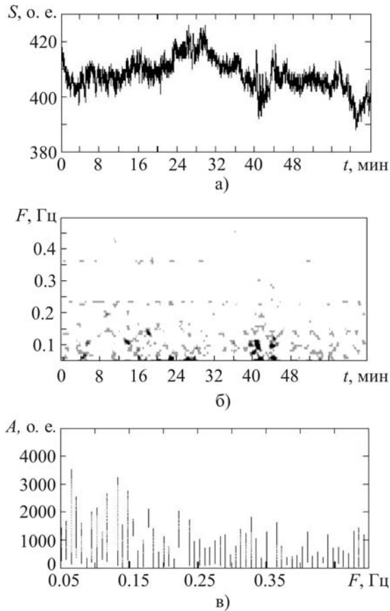
Рис. 6. Интенсивность излучения вспышки М6.1 12.09.2005г., начало записи в 08:48:12 UT, (а); спектрограмма флуктуаций излучения вспышки М6.1 12.09.2005 г. с началом в 08:48:12 UT (б); АЧХ пульсаций излучения вспышки М6.1 на временном интервале 08:55:42 UT \pm 1 мин (в)
