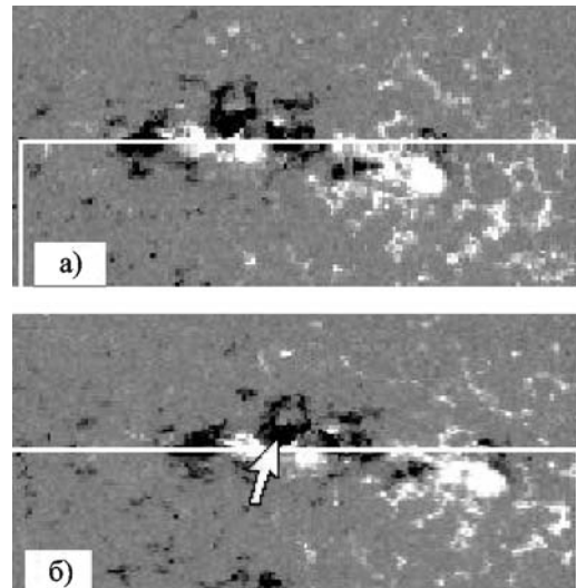
Рис. 2. Магнитограммы области NOAA9893 10.04.2002 г.: а) — для 04:48 UT; б) — для 12:48 UT. Стрелка — центр вспышки
