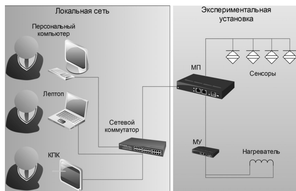
Рис. 5. Коллективное использование УПАК
