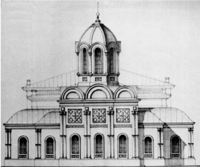
Рис. 6. Проект семінарської церкви архітектора Д. Арошина 1903 р.(південний фасад)
