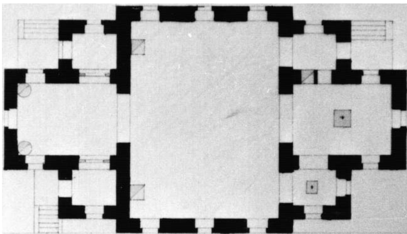
Рис. 5. Проект семінарської церкви архітектора Д. Арошина 1903 р. (план 1-го поверху)
