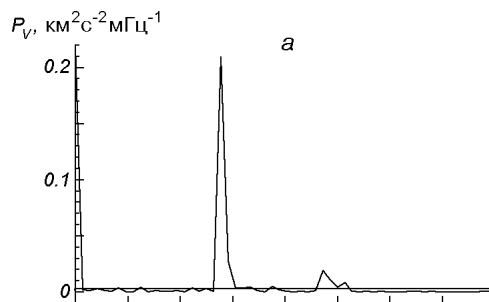
Рис. 7. Спектры мощности осцилляций скоростей V_z , флуктуаций газового давления \delta P и напряженности магнитного поля \delta B на уровне 1g\tau_5 = 0 . Прямой линией указан 99-процентный доверительный уровень, который определен согласно [23]
