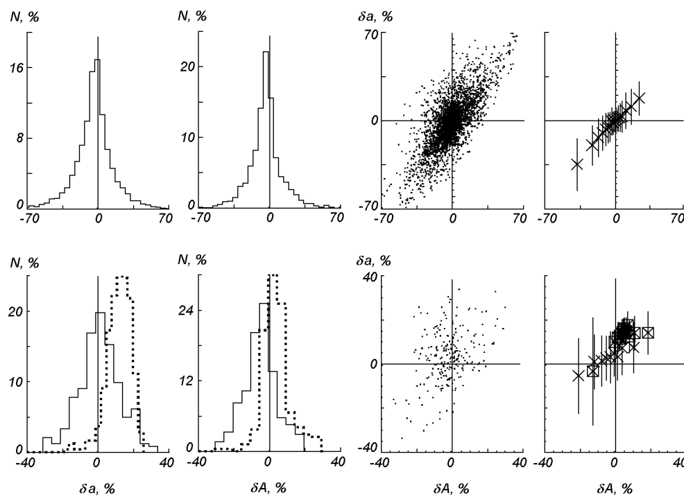
Рис. 8. Гистограммы распределений V -профилей по значениям параметров асимметрии амплитуд \delta a и площадей \delta A (средние значения соответственно \delta a = -1 , \delta A = -1 ), графики их рассеивания и их корреляционная связь: первый ряд — по всем анализируемым профилям, второй ряд — по усредненным (с шагом 700 км) профилям (средние значения \delta a = 3 , \delta A = -2 ). Пунктирная линия и квадратик — данные FTS-наблюдений
