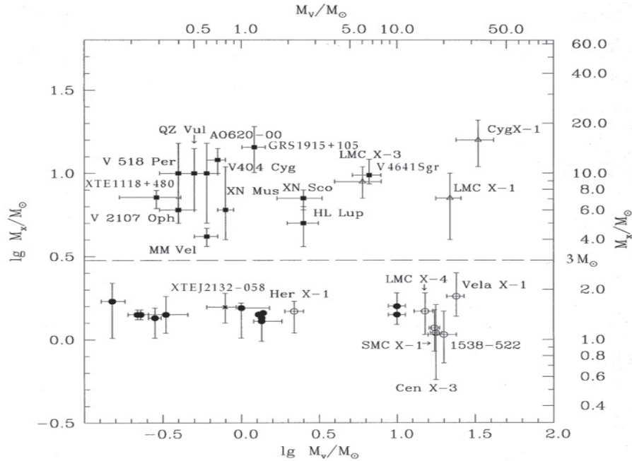
Рис. 1. Зависимость масс m_x н.з. (кружки и крестик) и ч.д. (треугольники и квадратики) от масс спутников m_v в тесных двойных системах (ТДС). Темные кружки соответствуют радиопульсарам, светлые кружки – рентгеновским пульсарам, крестик – н.з. в рентгеновской новой XTE J2132–058. Темные квадратики соответствуют ч.д. в рентгеновских новых, светлые треугольники – ч.д. в квазистационарных рентгеновских двойных системах с О–В компонентами
