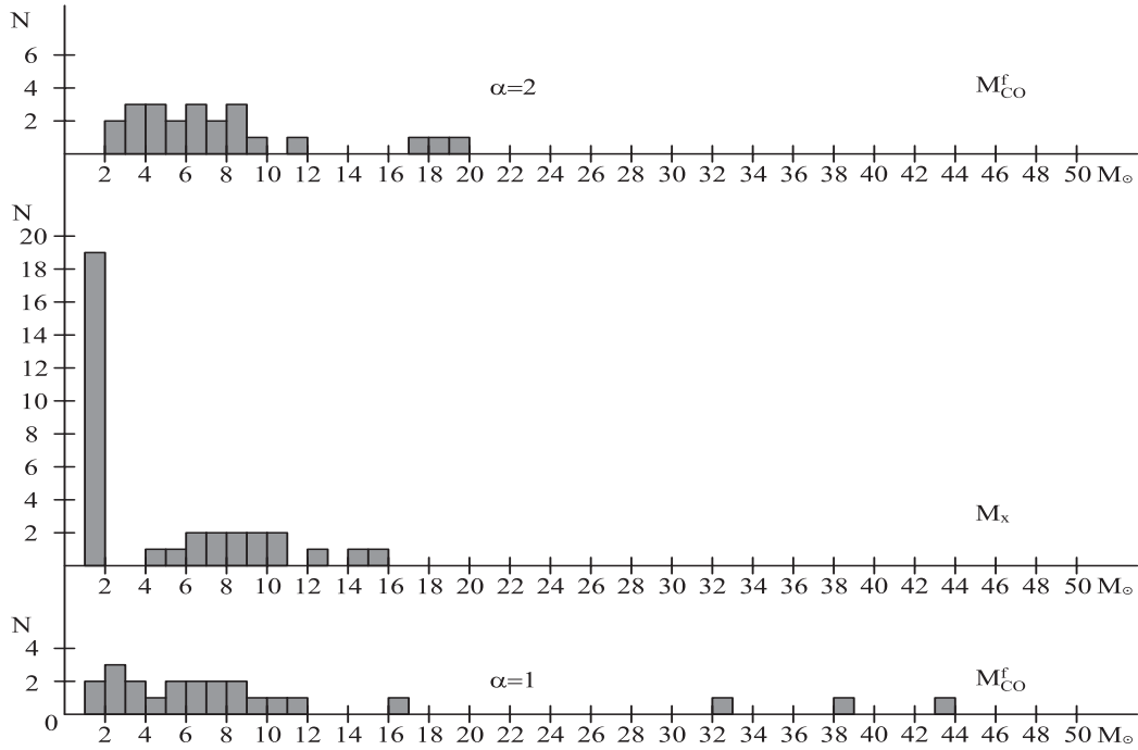
Рис. 2. Гистограммы распределения конечных масс углеродно-кислородных ядер M_{CO}^f для 23 звезд WR с известными массами (нижний график соответствует случаю \alpha = 1 в уравнении 2, верхний – случаю \alpha = 2 ). В середине показана гистограмма распределения масс M_x для 34 релятивистских объектов в ТДС. Высокий пик в диапазоне (1 - 2)M_\odot соответствует н.з. Распределения M_{CO}^f непрерывны, а распределение M_x бимодально с провалом в области значений масс M_x = (2 - 4)M_\odot
