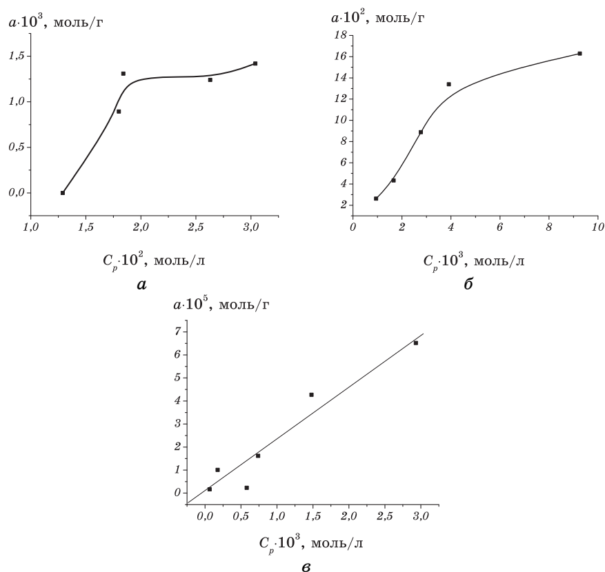
Рис. 3. Зависимость адсорбции пирокатехина (а), галловой (б) и кофейной (в) кислот на гидрофильной поверхности кремнезема А300; рН = 2.
