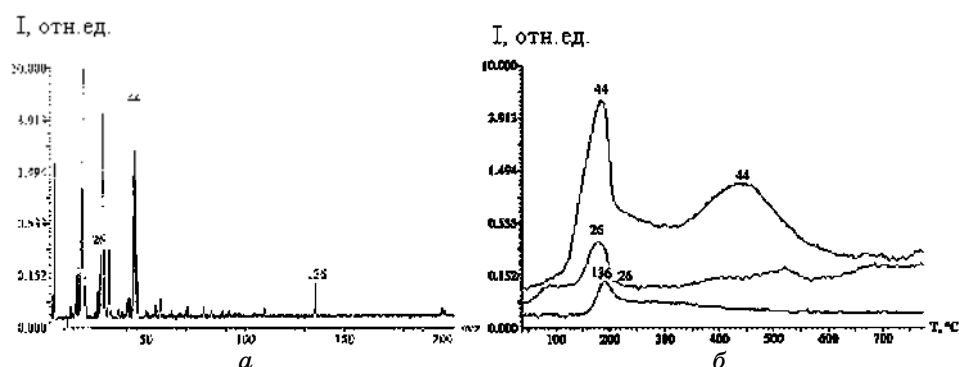
Рис. 7. Масс-спектр термического разложения при температуре (а) 463°C и термодесорбционные кривые (б) для 26, 44, 136 а.е.м. кофейной кислоты.
