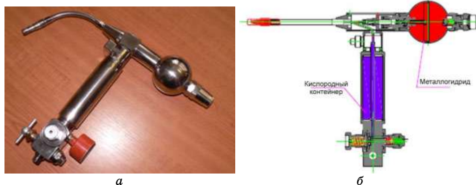
Рис. 8. Водородно-кислородная горелка с металлогидридным аккумулятором водорода, баллоном высокого давления для кислорода и пьезоэлектрическим поджигом факела.
