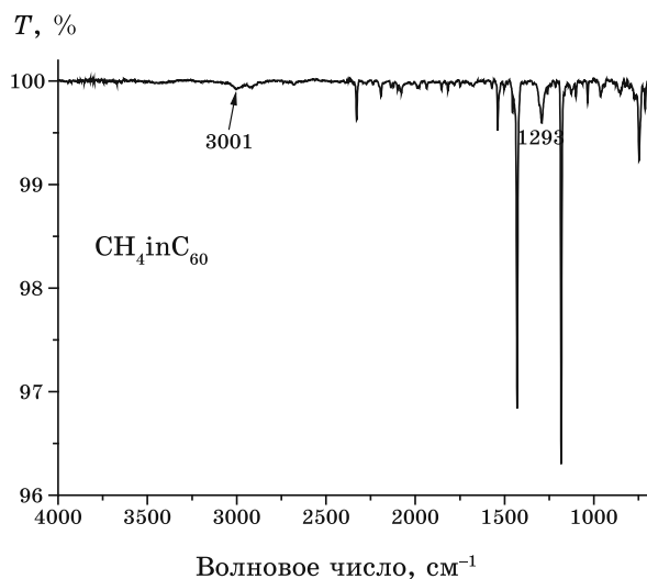
Рис. 1. ИК-спектр фуллерита (CH_4)_x C_{60} .
