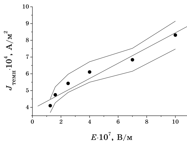
Рис. 4. Залежність темнового струму від прикладеного поля для зразка ПЕПК з 2,5 ваг. % \text{C}_{60} .
