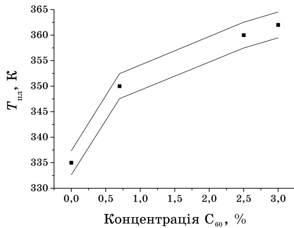
Рис. 9. Залежність температури переходу нанокмполитів ПЕПК-С 60 у в'язкоплинний стан від концентрації фуллеренів.
