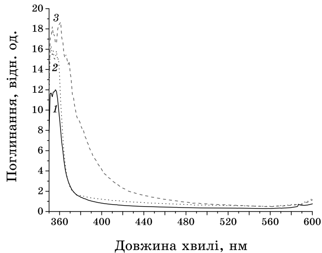
Рис. 2. Спектри вбирання политих зразків на кварці для ПЕПК (1), ПЕПК з 0,5 ваг.% С 60 (2) та ПЕПК з 3 ваг.% С 60 (3) (джерело випромінення — воднева лампа, температура — 300 К).
