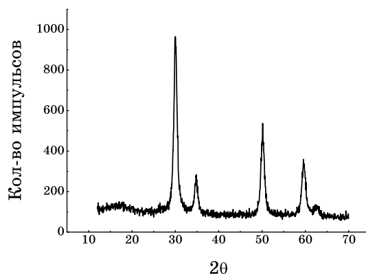
Рис. 2. Дифрактограмма образца диоксида циркония ( t -ZrO 2 ), полученного гидротермальным синтезом ( T = 250^{\circ}\text{C} , \tau = 6 час.) из продуктов разложения цирконового концентрата, содержащих в своем составе преимущественно фторцирконаты натрия.
