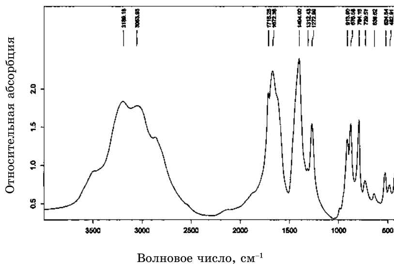
Рис. 3. Инфракрасный спектр сухого продукта.
