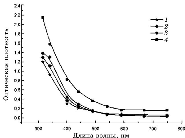
Рис. 1. Зависимость оптической плотности от длины волны падающего света для растворов, содержащих гидроксид аммония в объёме, мл: 1 — 1; 2 — 2,1; 3 — 8; 4 — расчётная зависимость.
