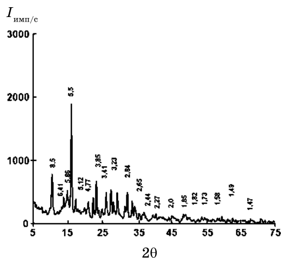
Рис. 2. Рентгеновская дифрактограмма нанодисперсного продукта.
