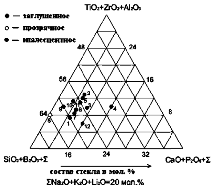
Рис. 1. Кристаллизационная способность исследуемых стекол в псевдотройной системе (\text{SiO}_2 + \text{B}_2\text{O}_3) + \Sigma - (\text{CaO} + \text{P}_2\text{O}_5) + \Sigma - (\text{TiO}_2 + \text{ZrO}_2 + \text{Al}_2\text{O}_3) , где \Sigma - (\text{Na}_2\text{O} + \text{Li}_2\text{O} + \text{K}_2\text{O}) .
