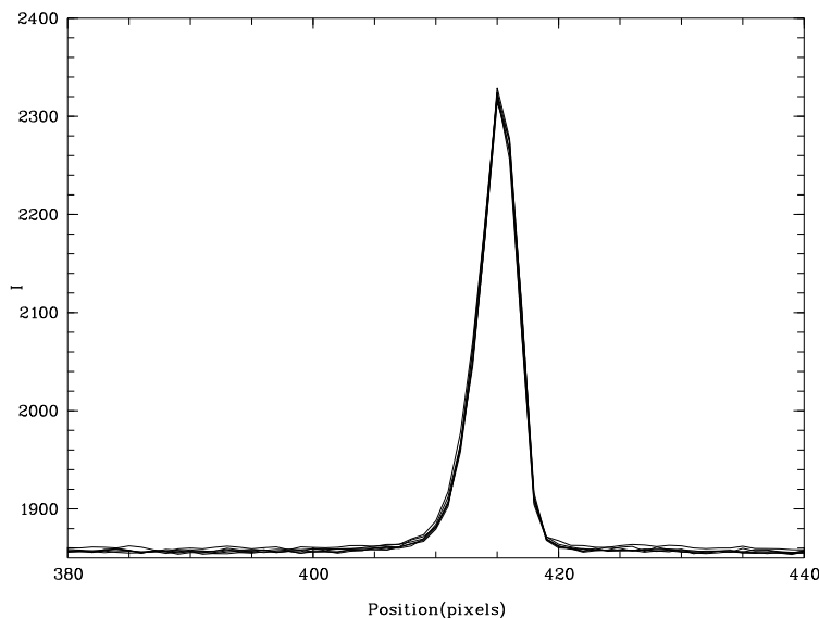
Рис. 6. Наложенные друг на друга спектры неона, полученные в течение ночи во время параллельных наблюдений на ОЗСП
