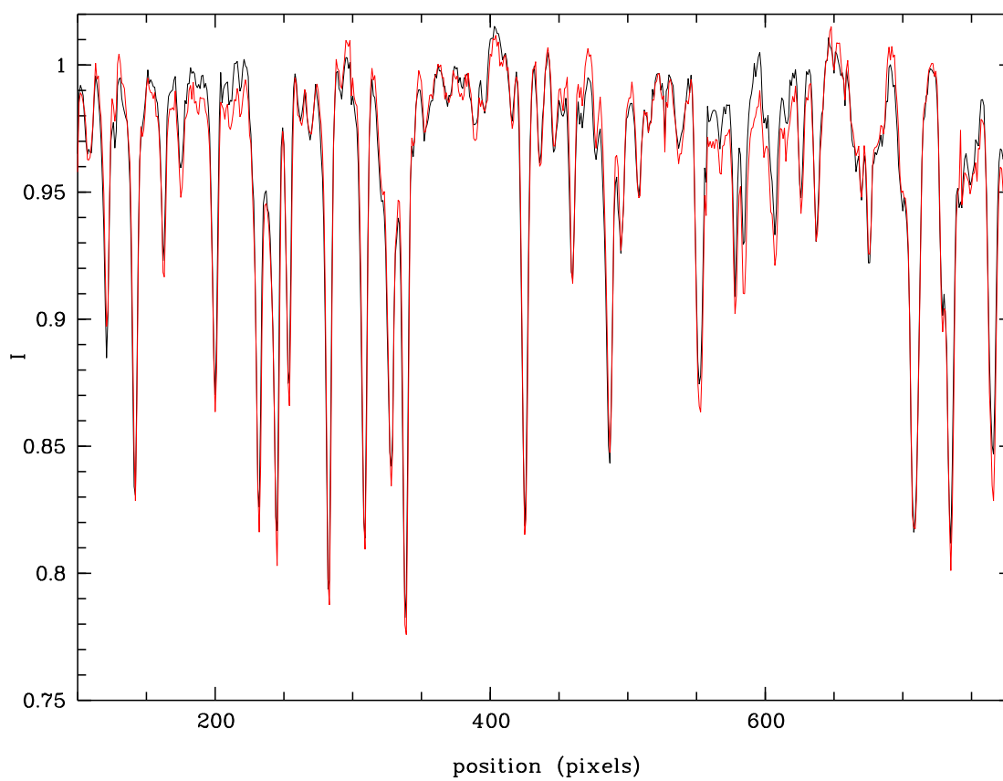
Рис. 5. Фрагмент экстрагированного 5-го порядка спектра \gamma Eri в двух поляризациях
