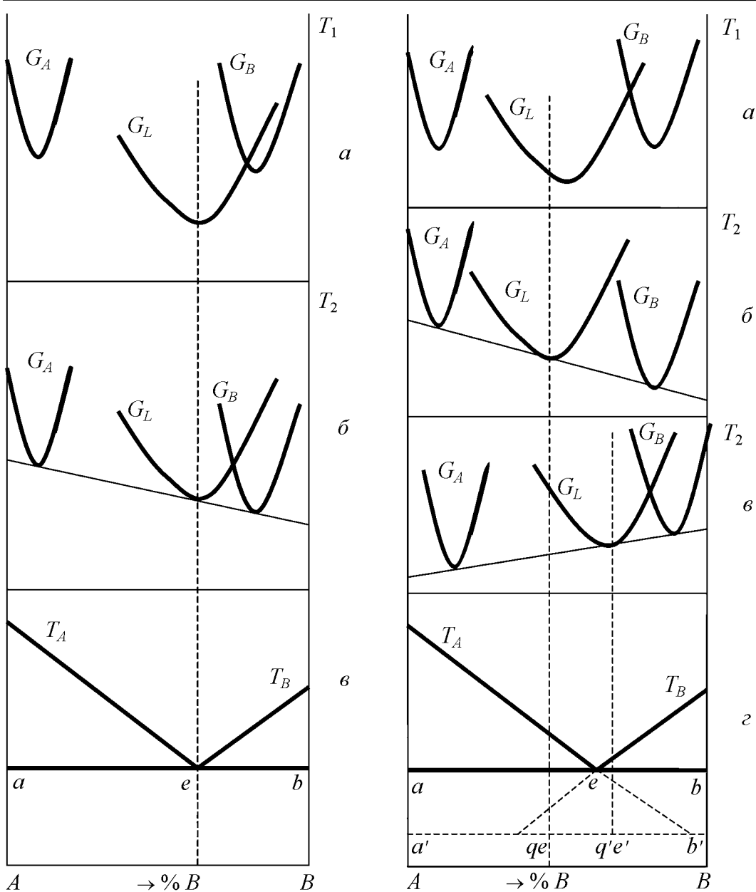
Рис. 1. Термодинамічні потенціали фаз ( a, б ) і відповідна евтектична діаграма стану ( в ) при відсутності розчинності в твердому стані
