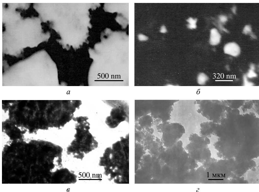
Рис. 1. Микрофотографии порошков: а и б – гидроксидов циркония и иттрия [9] ( а – агломераты, б – агрегаты); в – оксида циркония [10]; г – магнево-алюминиевой шпинели [11] (получены методом просвечивающей электронной микроскопии)
