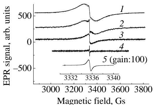
Рис. 3. ЭПР-спектры образца А1 на воздухе (кривая 1, n = 9 ) и при откачивании при T = 338 К на протяжении 0,5, 1, 2 и 4 h (кривые 2–5 соответственно). Амплитуда модуляции магнитного поля H_{\text{mod}} = 2,5, 1,25, 0,25, 0,025 и 0,0125 Gs для кривых 1–5 соответственно. Кривая 5 представлена в растянутом по H масштабе; пунктирная линия возле кривой 1 – аппроксимация (сумма двух лоренцевых линий); \nu = 9350 МГц
