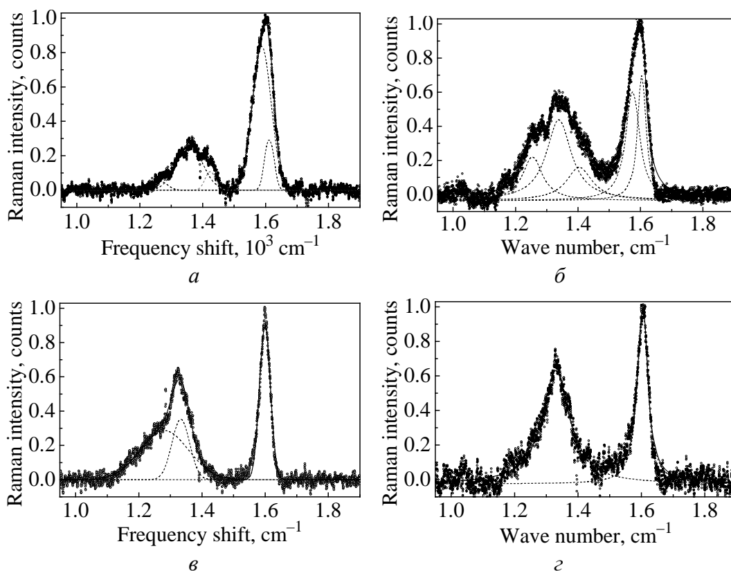
Рис. 5. КР-спектры углей разных марок: а – Д (шахта «Трудовская»), б – Ж (шахта им. А.А. Скочинского), в – А (шахта «2-2бис»), з – суперантрацит (шахта «Прогресс»)
