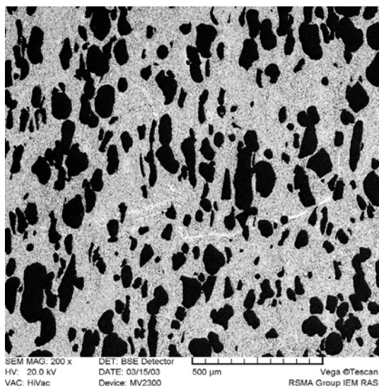
Рис. 1. Микроструктура спеченной контактной заготовки из сплава Cu–30% Cr
