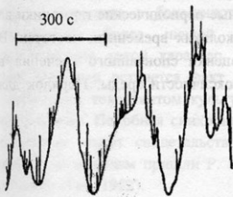
Рис. 3. Аналоговая запись осциллирующего спонтанного свечения Noctiluca scintillans Sur. (150 кл.).
