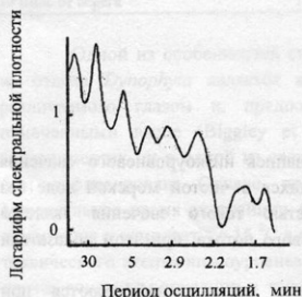
Рис. 4. Зависимость спектральной плотности излучений Noctiluca scintillans Sur. от периода осцилляций.
