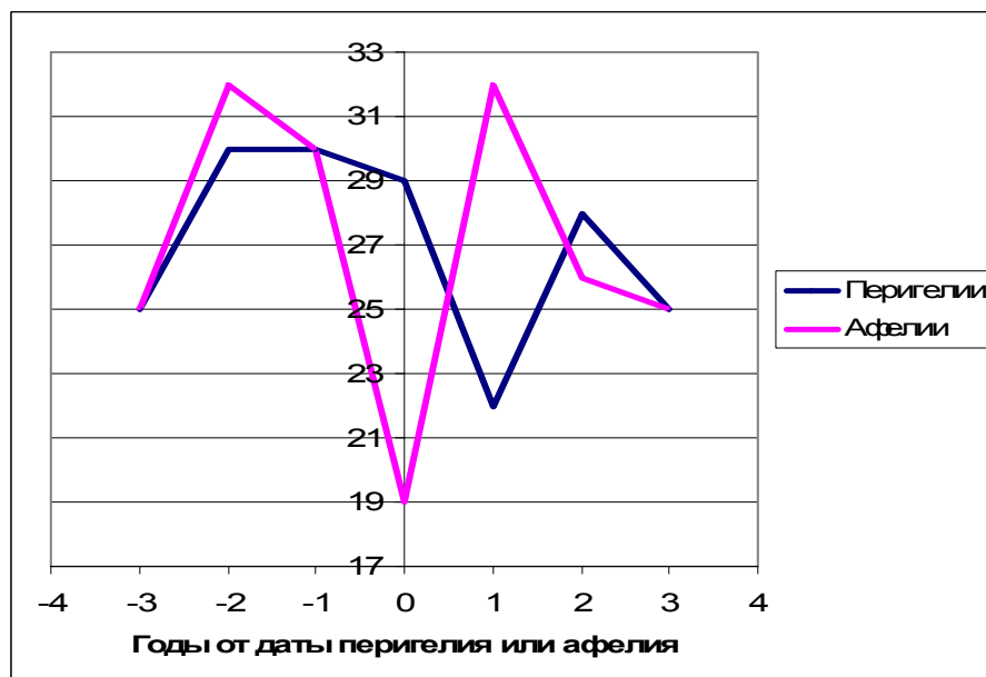
Рис. 9. Зависимость средней повторяемости зональной циркуляции в Северном полушарии Земли от орбитального движения Юпитера в период 1904-2006 гг. (9 циклов), дни
