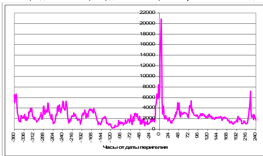
Рис. 5. Поток солнечного ветра во время прохождения перигелия Сатурном в июле 2003 г., протонов/кв. см в сек.
