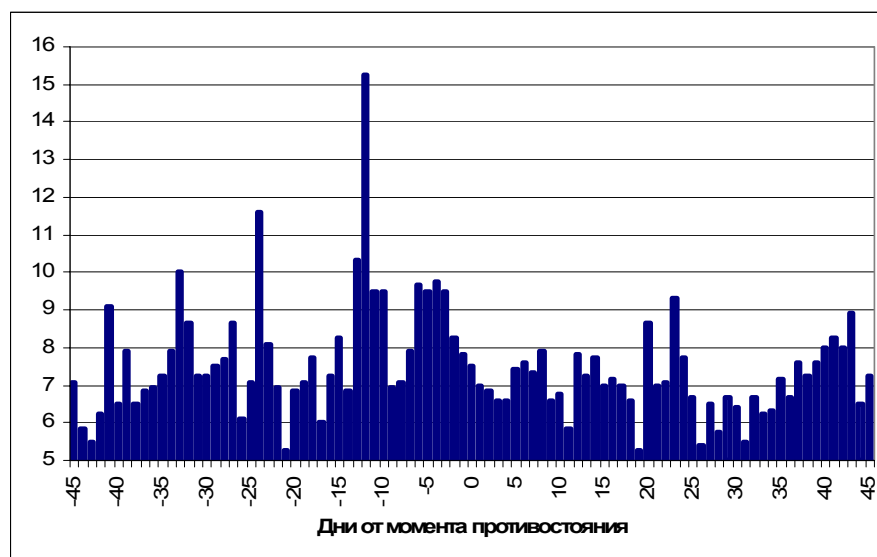
Рис. 27. Общее число землетрясений класса М5 за период 1998-2007 гг. в дни до и после противостояния Юпитера
