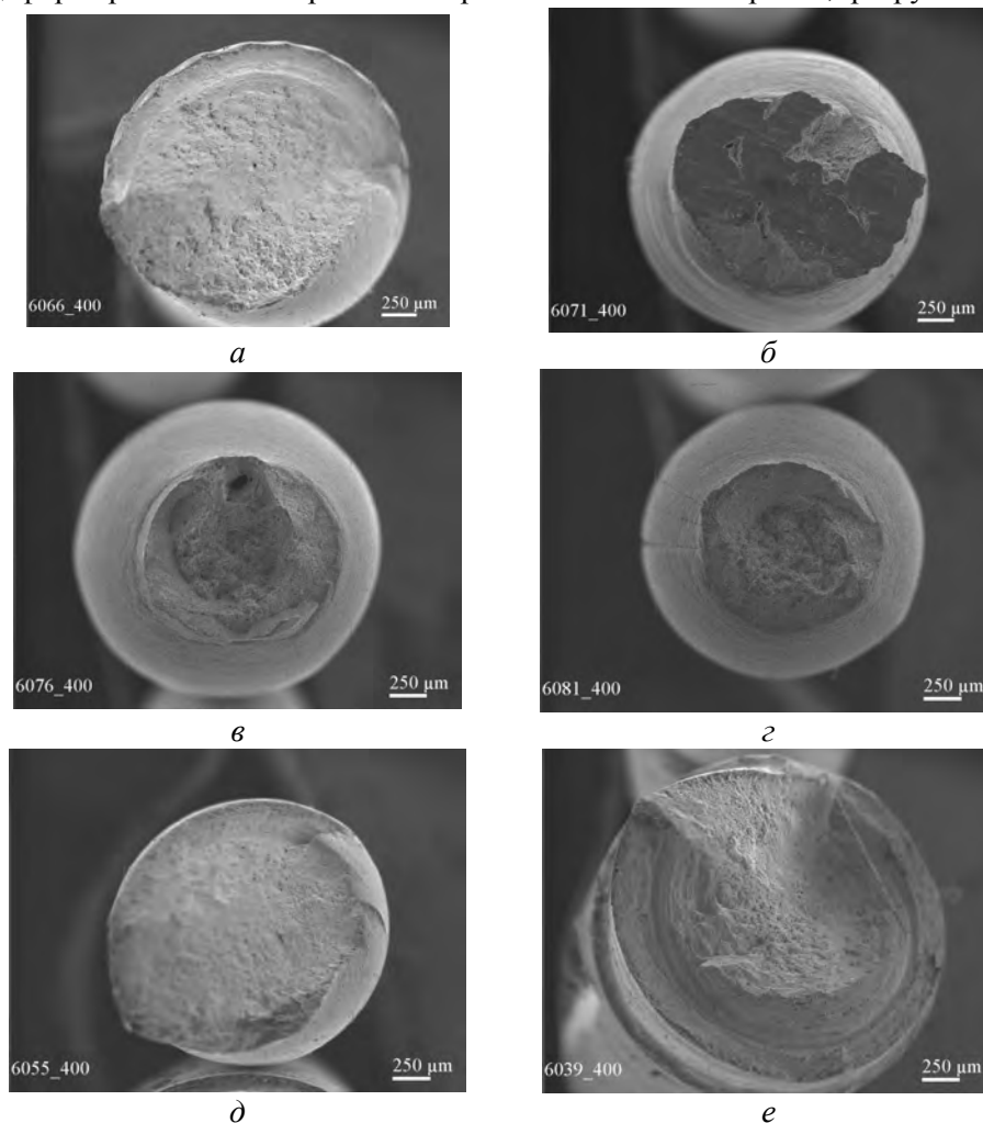
Рис. 5. Общий вид поверхности разрушения образцов, испытанных на одноосное растяжение после кручения на 25/0 (а), 25/10 (б), 25/15 (в), 25/25 (z), 25/50 (д) и 65/10 оборотов (е).
