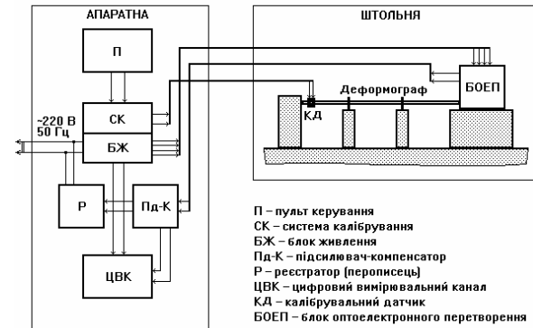
Рис. 2. Схема апаратурного комплексу кварцового деформографа з оптичелектронним вимірювальним каналом [Назаревич А., Назаревич Л., 2006]
