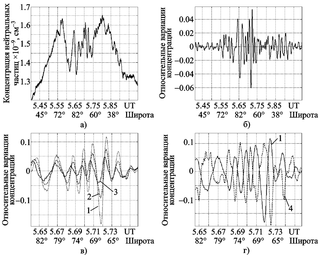
Рис. 1. Концентрации нейтральных частиц на витке 8296 в зависимости от инвариантной широты: а) – общая концентрация; б) – относительные вариации концентрации; в), г) – синхронные относительные вариации в разных сортах атмосферных газов (кривая 1 – Ar; кривая 2 – N_2 ; кривая 3 – O; кривая 4 – He). UT – всемирное время
