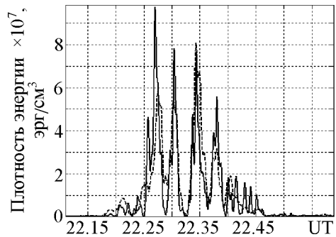
Рис. 3. Средние за период плотности кинетической E_K (штриховая кривая) и потенциальной E_p (сплошная кривая) энергии АГВ на витке 8132. Кинетическая энергия рассчитана по измерениям скорости нейтральных частиц в эксперименте WATS, потенциальная – по измерениям концентраций нейтральных компонент в эксперименте NACS на спутнике DE2
