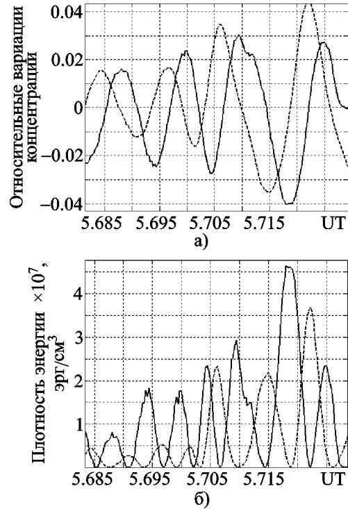
Рис. 2. Акустическая A (штриховая кривая) и гравитационная G (сплошная кривая) составляющие вариаций концентрации (а), распределения плотностей акустической E_A (штриховая кривая) и термобарической E_G (сплошная кривая) потенциальных энергий АГВ (б) на участке витка 8296
