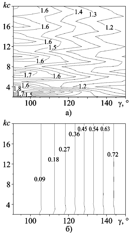
Рис. 5. Линии равных значений нормированного сопротивления излучения R кольцевого источника с kr_0 = 1 , \theta_0 = 5^\circ : а) – E -поляризация; б) – H -поляризация
