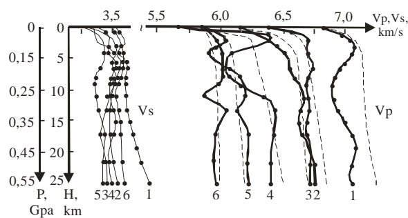
Рис. 2. Зміна V_{p,s}=f(P,T)=f(H) з глибиною для різних гранітоїдів:
