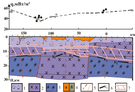
Рис. 3. Фрагмент схематичного розрізу речового складу земної кори ділянки геотраверса ІV:
