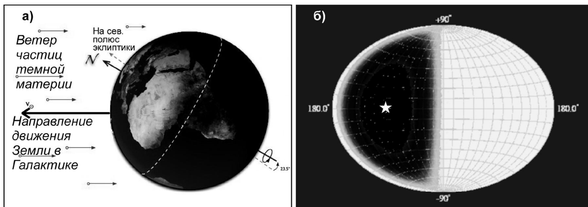
Рис. 1. Ветер частиц темной материи: а) Общая схема формирования ветра движением Земли в Галактике [36]; б) Корреляция распределения плотности потока частиц темной материи с движением Земли в Галактике [24]. Показана карта неба в галактических координатах. Меридианы – галактическая долгота, параллели – галактическая широта. Плоскость Галактики (Млечный путь) простирается вдоль экватора. Центральная точка – направление на центр Галактики. Звездочкой показано направление движения Земли в Галактике (направление на апекс). Заливкой (темным цветом) – распределение плотности потока частиц темной материи (данные численного моделирования)
