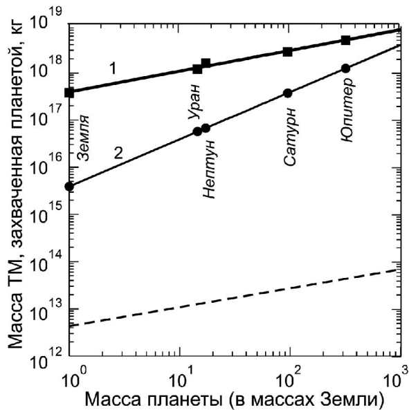
Рис. 6. Захват частиц темной материи планетами за время существования Солнечной системы. Верхние две зависимости – отображение результатов численного моделирования захвата: 1 – по [37], 2 – по [29]. Внизу – необходимое для обеспечения работы "космических печек" планет количество темной материи (в предположении аннигиляционного механизма тепловыделения и его постоянства во времени), по данным рис. 5, 6
