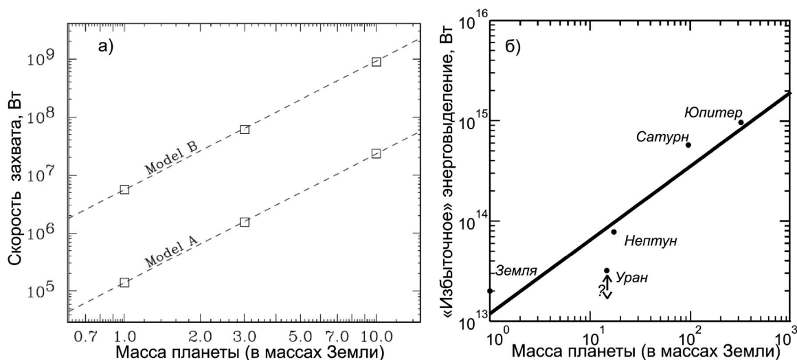
Рис. 5. Выделение "избыточной" (космической природы) энергии в недрах планет в зависимости от их массы: а) выраженные в единицах мощности расчетные значения скорости захвата и аннигиляции частиц темной материи, получаемые в результате численного моделирования для близких по составу к Земле планет (модели А и В различаются принятыми параметрами частиц) [27]; б) наблюдательные значения "избыточного" энерговыделения в недрах планет Солнечной системы [6]
