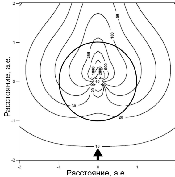
Рис. 4. Модельная плотность распределения атомов гелия межзвездной среды в Солнечной системе (в плоскости, содержащей ось ветра) [32]. Солнце находится в центре системы координат, расстояния даны в астрономических единицах. Окружность – орбита Земли. Стрелка – ось межзвездного гелиевого ветра. Изолиниями показано соотношение локальной плотности к фоновой плотности за пределами Солнечной системы. Фокусирующий конус (focusing cone) формируется за Солнцем с тыльной стороны. Полость на наветренной стороне – результат процессов ионизации
