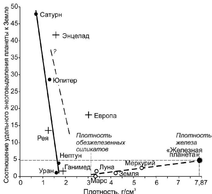
Рис. 7. Соотношение выделения "избыточной" (не радиогенной) энергии на единицу массы в недрах планет по отношению к Земле в зависимости от их плотности (с вычетом гравитационного сжатия для планет земной группы) [6]
