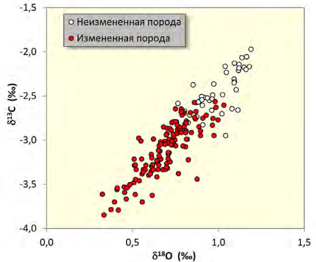
Рис. 6. Отношение значений \delta^{13}\text{C} и \delta^{18}\text{O} неизмененных и слабо измененных палеоценовых известняков у с. Скалистое.
