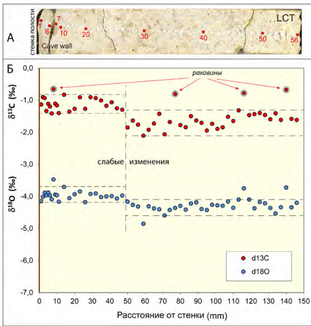
Рис. 13. Фото образца LCT из пещеры Подарочная (А) и изменение изотопного состава по профилю керна (Б). Керн пробурен в стенке карстовой полости через вмещающую породу. Длина керна около 145 мм.
