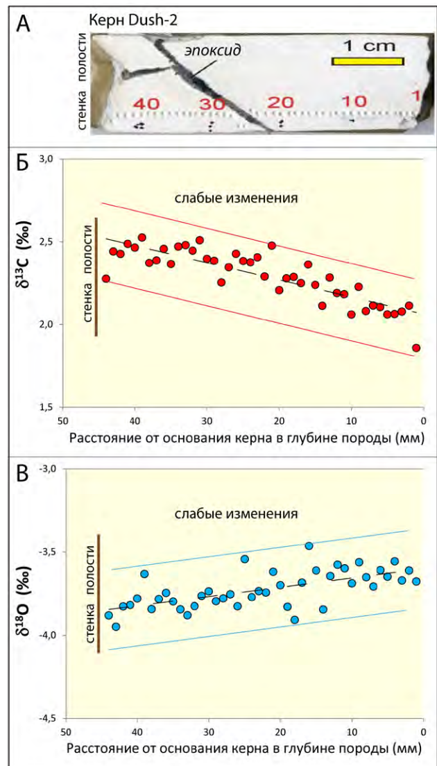
Рис. 17. Фото образца Dush-2 из пещеры Душевского (А) и изменение изотопного состава углерода (Б) и кислорода (В) по профилю керна. Керн пробурен в стенке карстовой полости. Шаг опробования на профиле 1 мм. Штриховыми линиями обозначены тренды по рядам данных, сплошными линиями – коридоры значений.
