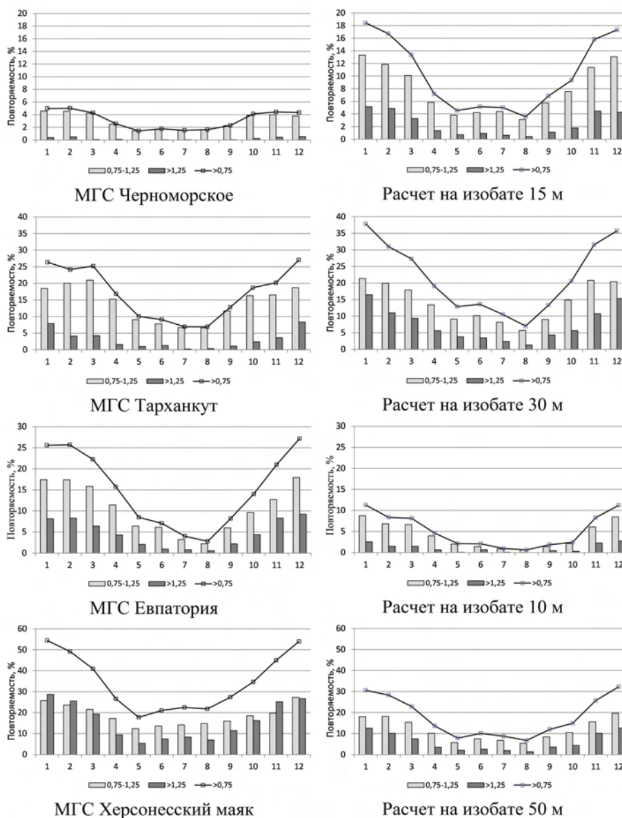
Р и с . 2 . Повторяемость (%) различных градаций высот волн (м) по месяцам на береговых станциях и по данным ре-анализа. Градации волн выбраны на основании стандартной шкалы степени волнения и соответствуют баллам волнения.
