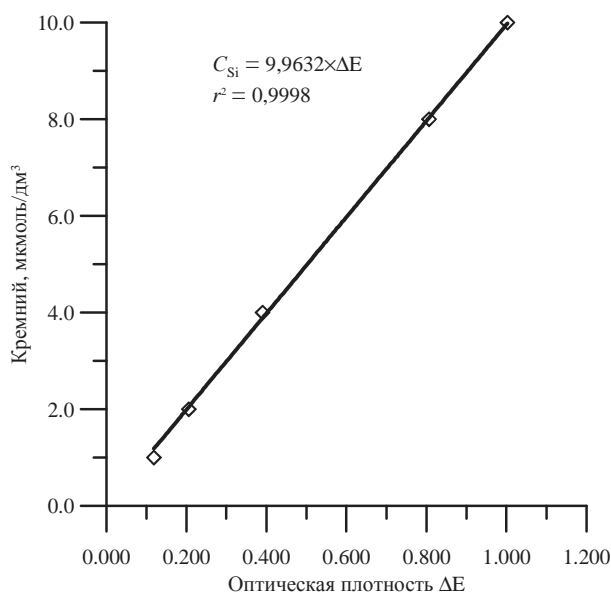
Р и с. 2. График градуировочной зависимости концентрации кремния C_{Si} в морской воде от оптической плотности \Delta E
